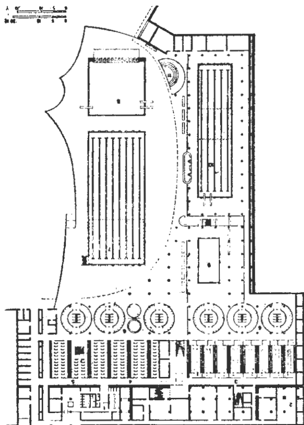
En skiss över olympiska badet i München. Damerna har 4 omklädningsrum — herrarna har 5. På bilden syns tävlings-, hopp- och träningsbassäng. Åskådarp plats för 10.000.
